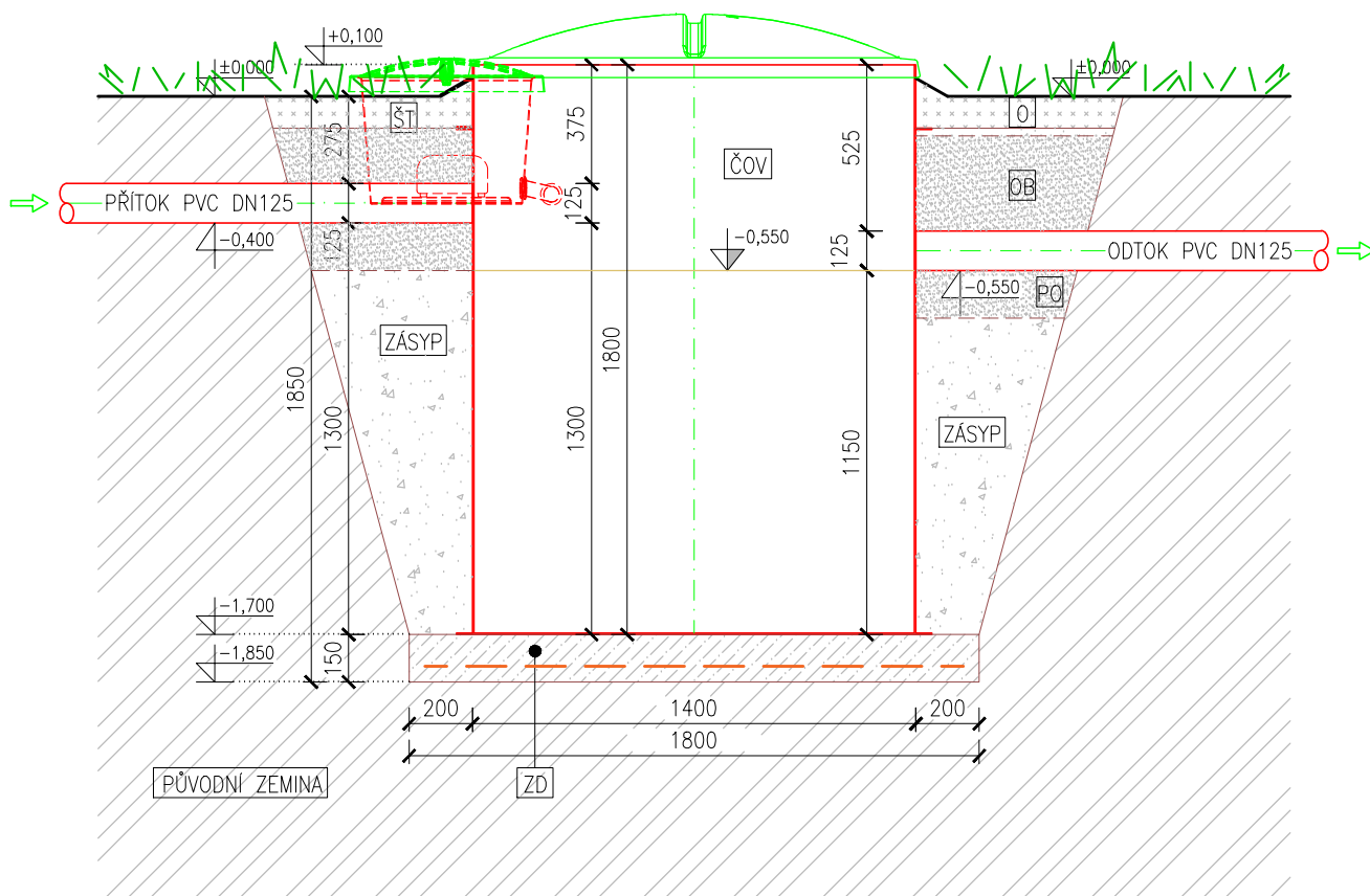
ŘEZ - OSAZENÍ
